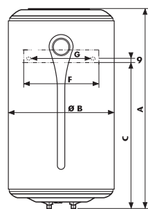
Вид спереди
